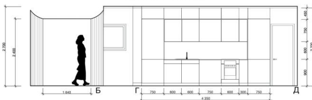
РОЗГОРТКИ СТІН 1:25
